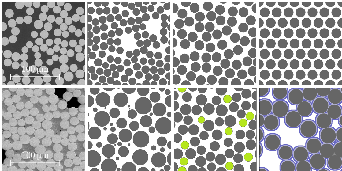
FIGURE 3.1 – Sections transverses de matériaux composites unidirectionnels réels (avec barre d'échelle) et virtuels. La répartition spatiale des fibres est souvent très hétérogène et ces fluctuations morphologiques induisent des comportements qu'il est parfois difficile d'appréhender par des tests physiques. Les outils numériques permettent de modéliser des configurations virtuelles plus ou moins complexes pour explorer les propriétés de microstructures représentatives. D'après POULET (2017).
