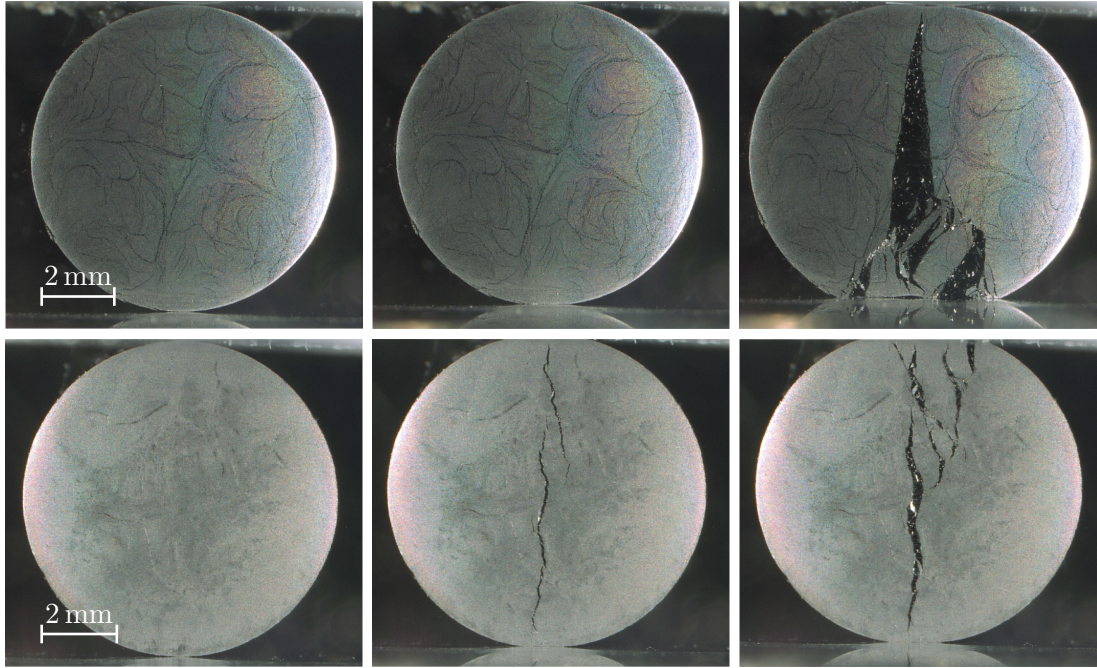
FIGURE 3.7 – Prise d’images à différents chargements en compression diamétrale de deux jones composites ( \varnothing 8 mm) de natures différentes : carbone/époxy en haut et verre/polyamide en bas. D’après CAYZAC (2014).
