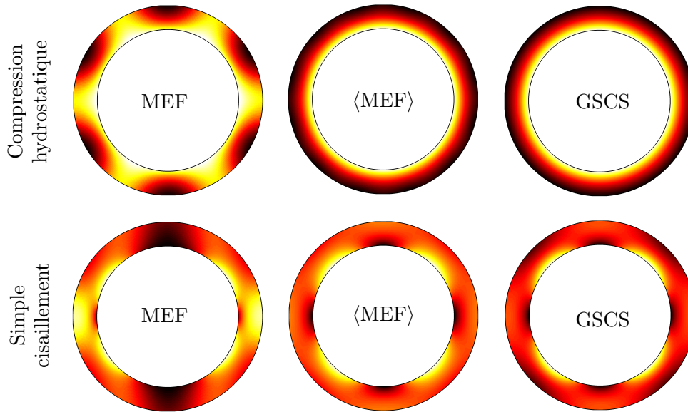
FIGURE 5.1 – Comparaison des champs locaux entre un arrangement hexagonal (MEF) et les résultats obtenus par la méthode autocohérente généralisée (GSCS). Un post-traitement appliqué sur les résultats numériques ( \langle \text{MEF} \rangle ) permet de retrouver les résultats GSCS à l'interface fibre/matrice.
