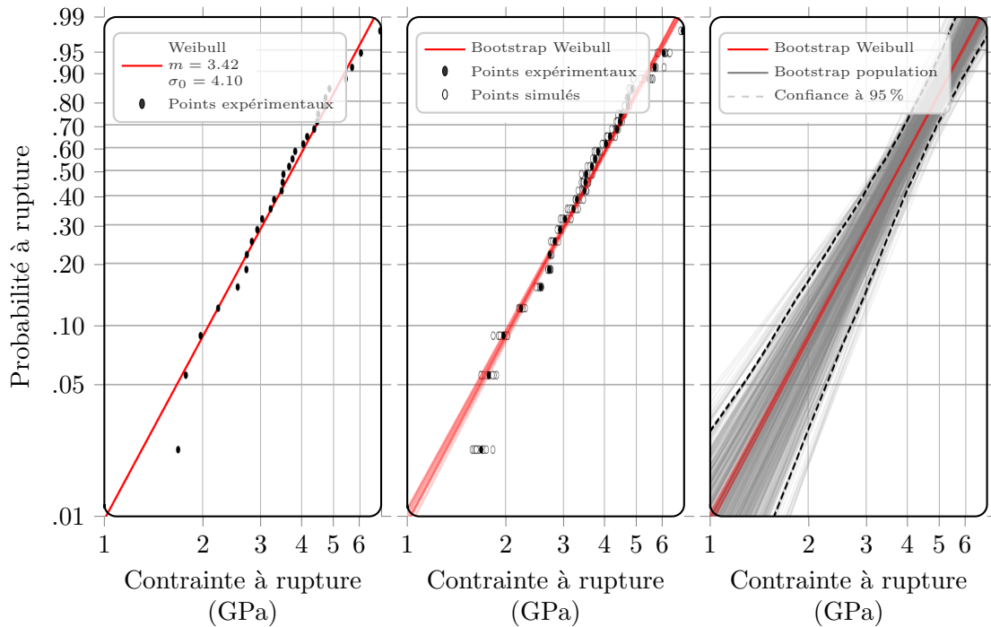
FIGURE 4.9 – Probabilités à rupture cumulées pour un jeu de 30 tractions sur monofilaments de 30 mm de longueur. Le graphique de gauche est celui habituellement rapporté dans la littérature. Celui du centre prend en compte l’incertitude expérimentale et celui de droite l’incertitude liée à la taille de l’échantillon (JOANNÈS, ISLAM et LAIARINANDRASANA, 2020).
