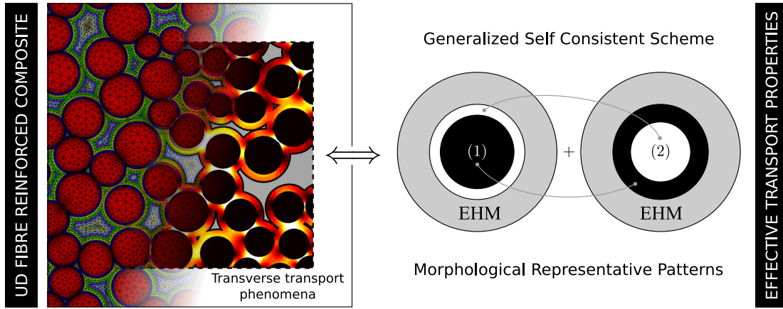
FIGURE 3.13 – Le milieu composite (à gauche) est modélisé par une approche à 2 phases - 2 motifs (à droite) enveloppées dans le milieu homogène équivalent. Sur l'image de gauche, la norme du flux est représentée par un gradient de couleur allant du jaune pâle au noir (flux nul). Les zones grisées correspondent aux zones de matrice « piégée » (JOANNÈS et HERVÉ-LUANCO, 2016).
