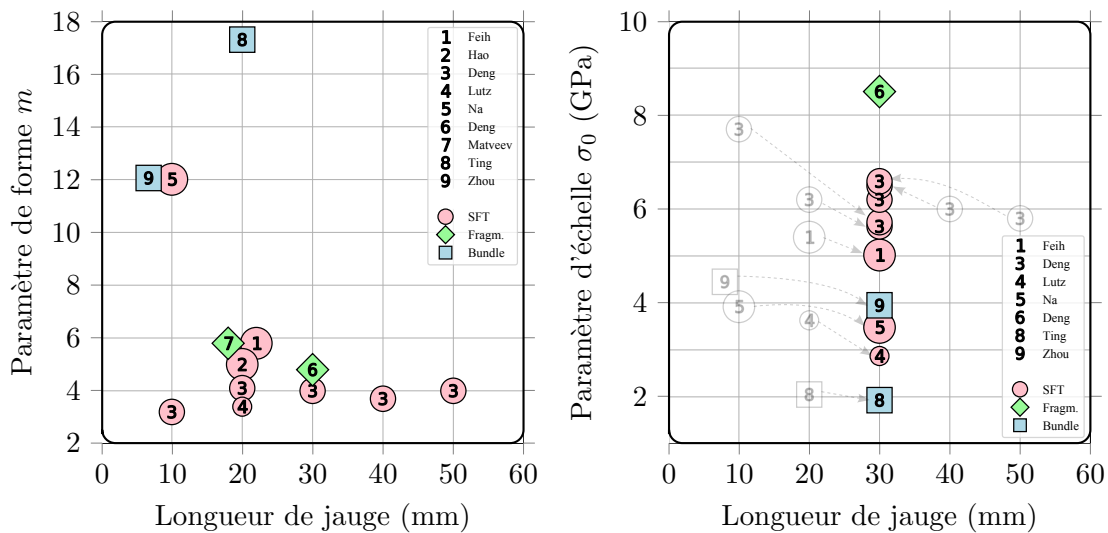
FIGURE 4.7 – Valeurs des paramètres de Weibull pour les fibres de carbone T700 publiées dans la littérature. Se référer à JOANNÈS, ISLAM et LAIARINANDRASANA (2020) pour les références concernées. Les marqueurs en forme de cercle, de losange et de carré représentent respectivement les résultats des essais en traction sur fibres individuelles, des essais de multi-fragmentation et des essais sur mèches. La taille des cercles est proportionnelle à la taille de l'échantillon testé. Les valeurs du paramètre d'échelle ont été normalisées pour une longueur de jauge de 30 mm.
