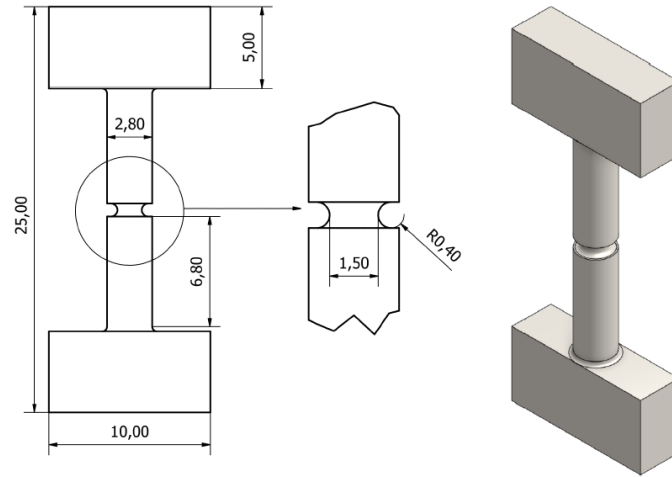
FIGURE 3.9 – Mini-éprouvette de laboratoire entaillée destinée à concentrer la triaxialité des contraintes à cœur. Les cotes sont indiquées en millimètres (POULET, 2017).
