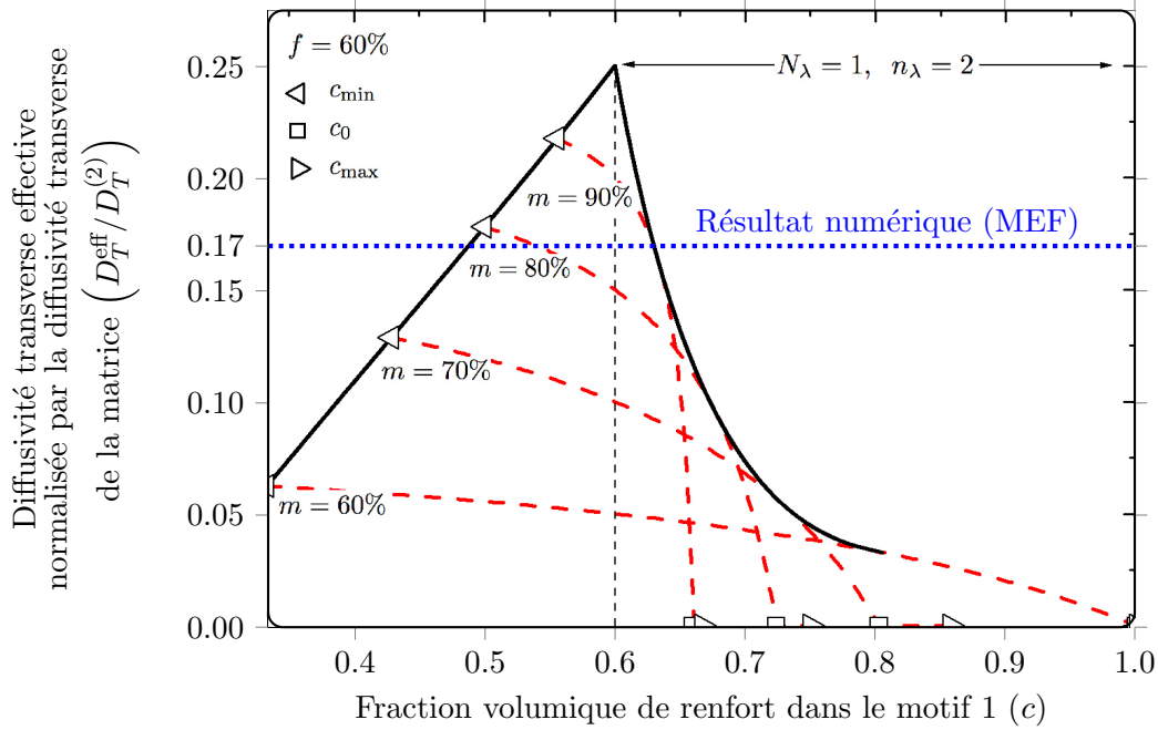
FIGURE 3.14 – Courbe enveloppe de la diffusivité effective transverse D_T^{\text{eff}} normalisée par la diffusivité de la phase (2) (matrice). La fraction de renfort est fixée à 60% et le paramètre c est borné tel que 0 \leq c_{\min} = 1 + (f - 1)/m < c < c_{\max} = f/m \leq 1 . Puisque D_T^{(1)} = 0 dans le cas considéré, nous pouvons faire apparaître un paramètre c_0 tel que pour c_0 < c < c_{\max} , D_T^{\text{eff}} = 0 . Nous avons par ailleurs m \geq 1/2 + |f - 1/2| . Le « sommet » de la courbe enveloppe correspond au modèle GSCS à trois phases classique (JOANNÈS et HERVÉ-LUANCO, 2016).
