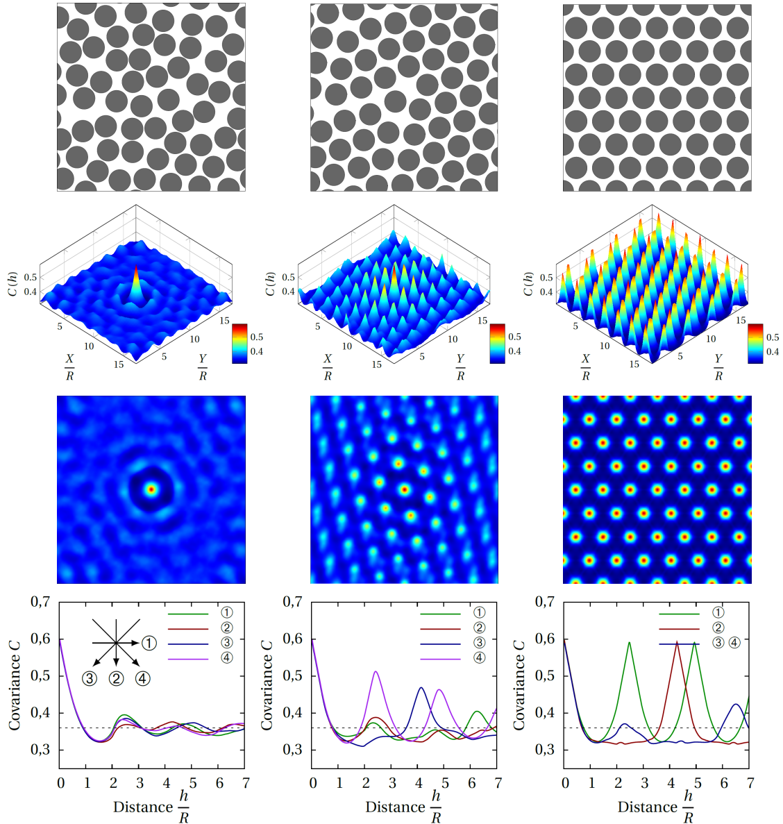
FIGURE 3.5 – Illustration de la covariance pour trois microstructures présentant la même fraction surfacique/volumique de renfort mais des distributions plus ou moins aléatoires. Les covariogrammes 3D et 2D sont représentés sur les 2 ème et 3 ème lignes. La 4 ème ligne correspond aux fonctions de covariance suivant quatre directions différentes. Tant le caractère aléatoire que le caractère périodique des microstructures, respectivement à gauche et à droite de la figure, apparaissent clairement (POULET, 2017).
