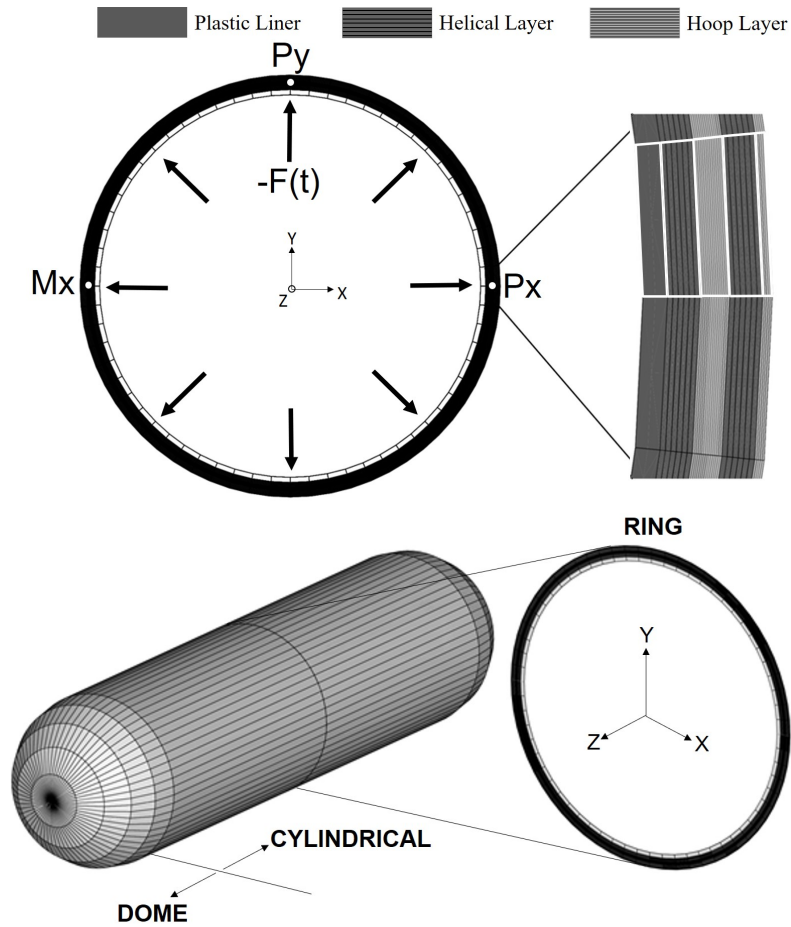
FIGURE 2.14 – Illustration du concept SERFAIR appliqué à un domaine annulaire sur un réservoir type IV de 6.8L. Le maillage dans l’anneau, statistiquement représentatif, présente les caractéristiques nécessaires pour rendre compte des mécanismes d’endommagement décrits dans ce chapitre. Le maillage extérieur au domaine est quant à lui plus grossier. D’après (WIDJAJA, 2020).
