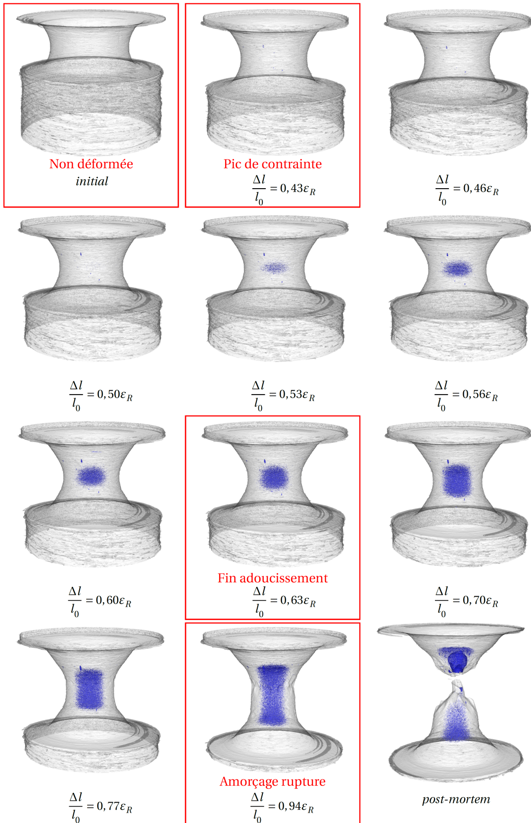
FIGURE 3.11 – Mise en évidence, par reconstruction tomographique puis segmentation, de l'évolution des cavités (en bleu) au droit de l'entaille (rayon initial de 400\ \mu\text{m} ) de l'éprouvette Bulky au cours de l'essai de traction. Les valeurs des paliers de déplacement sont indiqués sous chaque sous-figure. D'après POULET (2017).
