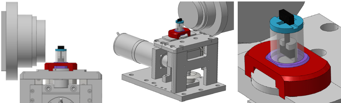
FIGURE 3.10 – Machine Bulky : dispositif expérimental pour le suivi in situ de l'essai de traction. L'éprouvette, est ici représenté en noir, est installé dans les mors et est visible à travers le tube de PMMA (POULET, 2017).
