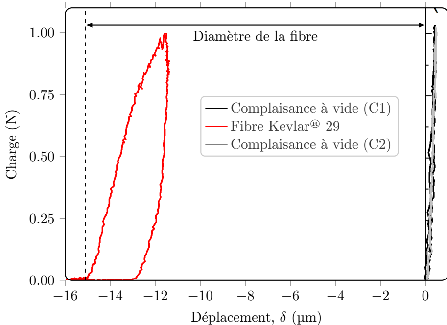
FIGURE 4.5 – Protocole expérimental pour la compression diamétrale : premier test de complaisance (C1) à vide, compression de la fibre puis second test de complaisance (C2) à vide.
