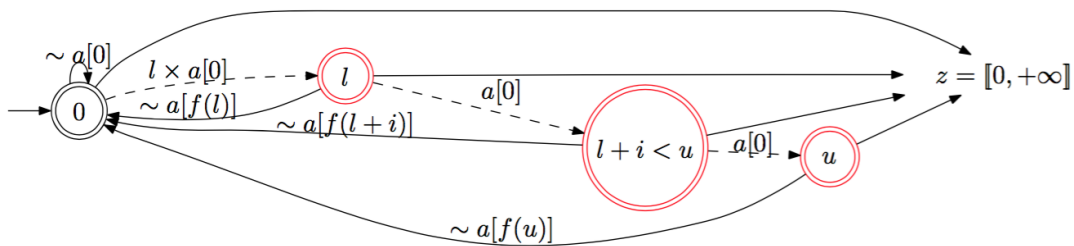
FIGURE 2.12 – Automate autorisant uniquement les stretches de a de longueur l + i avec i compris entre 0 et u - l et associant une pénalité fonction de cette longueur f(l + i) .
