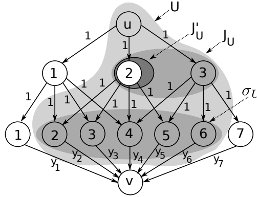
FIGURE 2.3 – Le graphe du modèle de flot pour 3 variables, 7 valeurs et un exemple de coupe, U en gris clair, les ensembles de noeuds J \cap U et \Sigma \cap U en gris moyen, et J'_U in gris foncé.
