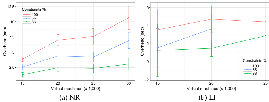
FIGURE 2.2 – Impact des contraintes utilisateur sur les temps de résolution sur les instances NR (gauche) et LI (droite)
