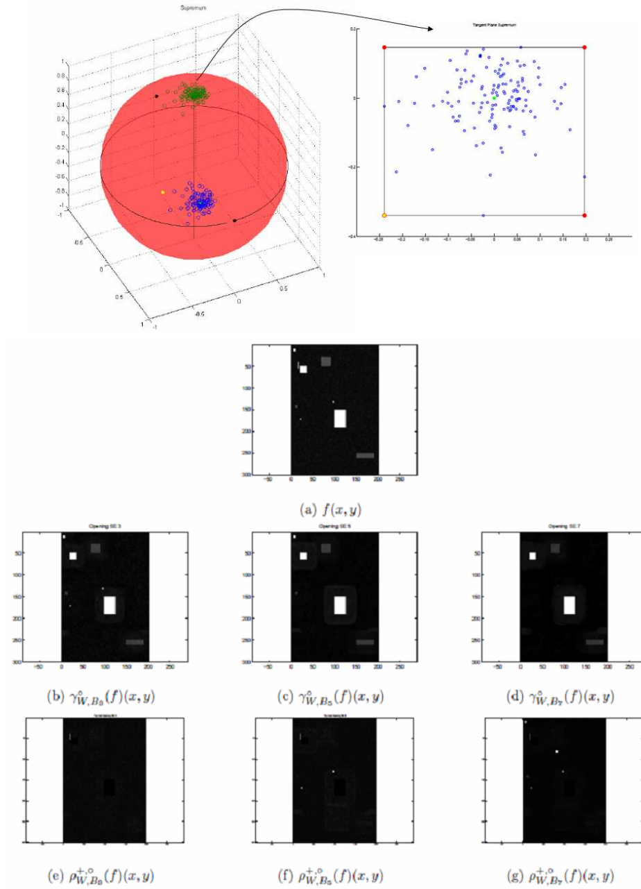
FIG. 7.3 – Morphologie mathématique sur la sphère S^2 : haut, origine locale sur la sphère et calcul du sup/inf sur l'espace tangent ; bas, application des résidus d'ouvertures sur la sphère pour la détection de cibles sur des images Radar polarimétriques.
