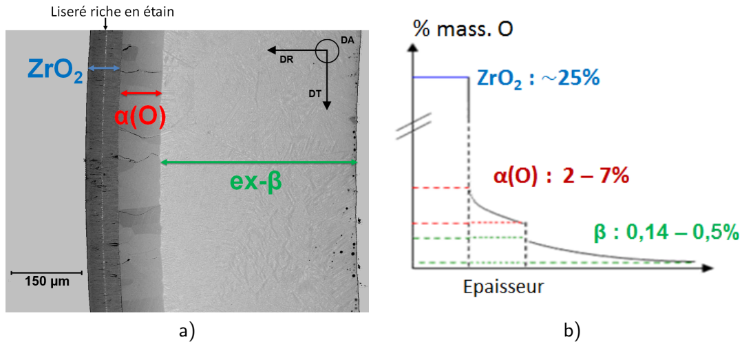
FIGURE I.21 – Microstructure d'une gaine oxydée à haute température et schéma du profil de la concentration en oxygène — micrographie MEB sur Zircaloy-4 oxydé sous vapeur 520 s à 1200 °C [101].
