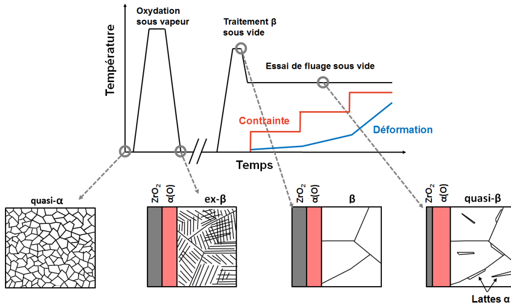
FIGURE II.56 – Schéma du cycle thermo-mécanique de l’essai de fluage axial sous vide sur gaine en M5 ® pré-oxydée sous vapeur à haute température ; microstructures schématiques de la gaine aux différentes étapes de l’essai (peau externe à gauche).
