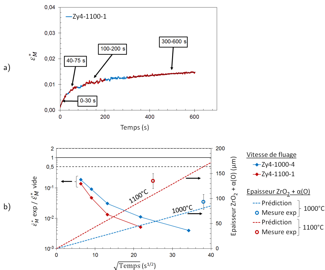
FIGURE III.57 – a) déformation vraie équivalente \epsilon_M^* en fonction du temps. Essai de fluage (Zy4-1100-1) à 1100 °C, sous 5 bar ( \sigma_M^* = 2,8 MPa) de pression interne et sous vapeur sur Zircaloy-4 et b) évolution en fonction du temps de l'accord vide/vapeur (à partir de la loi de fluage sous vide identifiée par Fréchet [1]) et de l'épaisseur cumulée de zircone et de phase \alpha(O) (d'après les données DEZIROX + CINOG BP [117]) — Zircaloy-4, domaine \beta .
