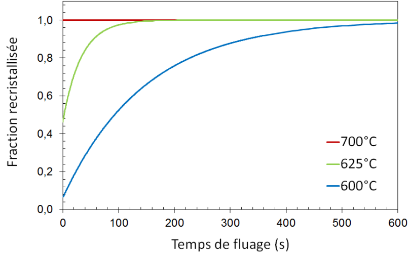
FIGURE II.26 – Évolution de la fraction de matière recristallisée dans le Zircaloy-4 pendant l’essai de fluage, après une rampe à 25\text{ °C s}^{-1} et un maintien de 20 s à la température de fluage avant mise sous pression, d’après le modèle de Sills et Holt [149].
