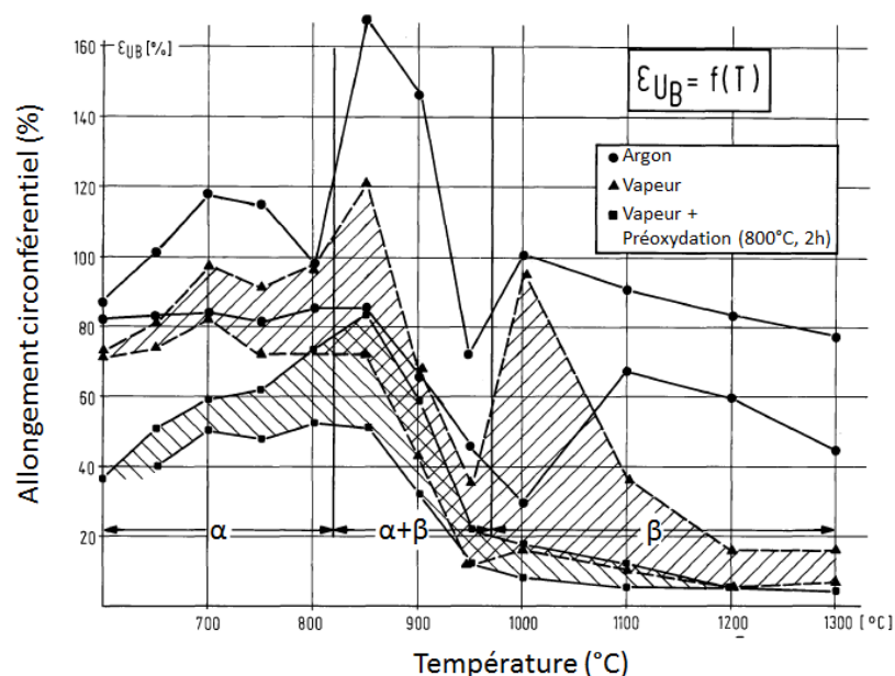
FIGURE II.22 – Évolution de l'allongement circonférentiel à rupture en fonction de la température — Essais de fluage sur gaine en Zircaloy-4 sous pression interne dans une atmosphère d'argon, d'air ou de vapeur, avec ou sans pré-oxydation sous vapeur à 800 °C pendant 2 h, d'après [190].
