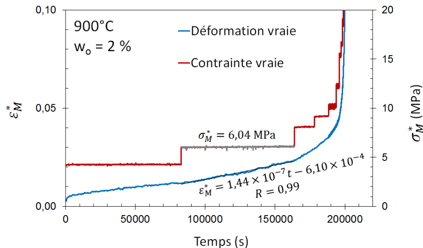
FIGURE III.39 – Déformation vraie équivalente \epsilon_M^* et contrainte vraie équivalente \sigma_M^* en fonction du temps. Essai de fluage axial sous vide à 900 °C sur gaine « modèle » base M5® contenant 2 % en masse d'oxygène.
