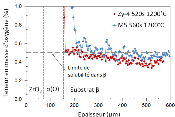
FIGURE III.3 – Profils de diffusion de l'oxygène, mesurés par microsonde, dans les épaisseurs de gaines en Zircaloy-4 et en M5® oxydées à 1200 °C sous vapeur [120]. Les interfaces pour le Zircaloy-4 sont repérées en pointillés.
