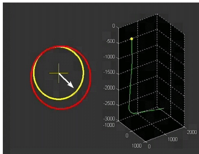
FIG. 3 – Visualisation 3D par ABIS de la position et de la force de contact latéral entre la garniture et la paroi du puits de forage
