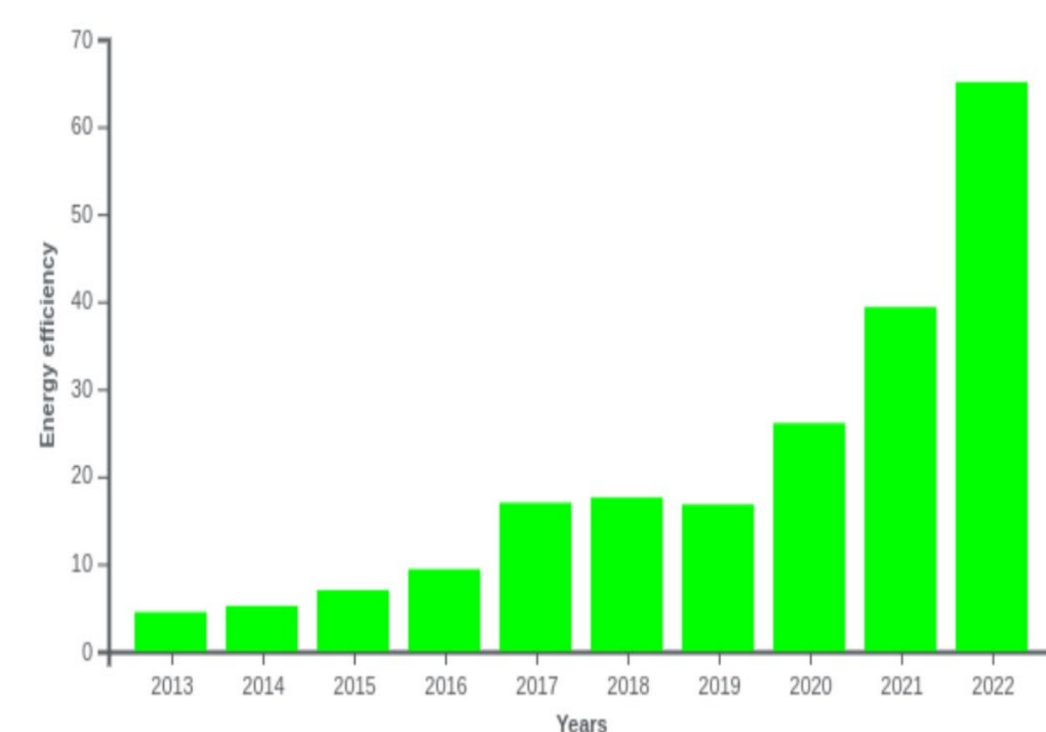
Amélioration de l'efficacité énergétique des supercalculateurs du Green500.[2]
