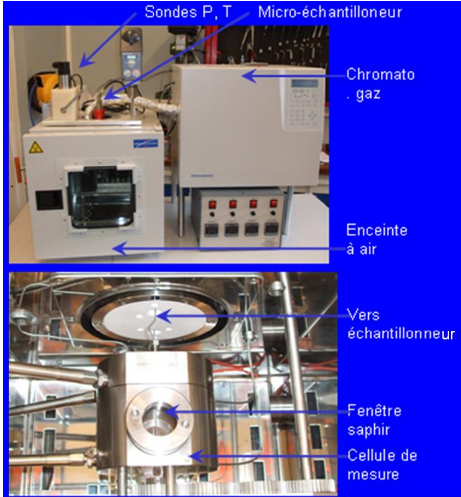
Dissolution à l'équilibre
