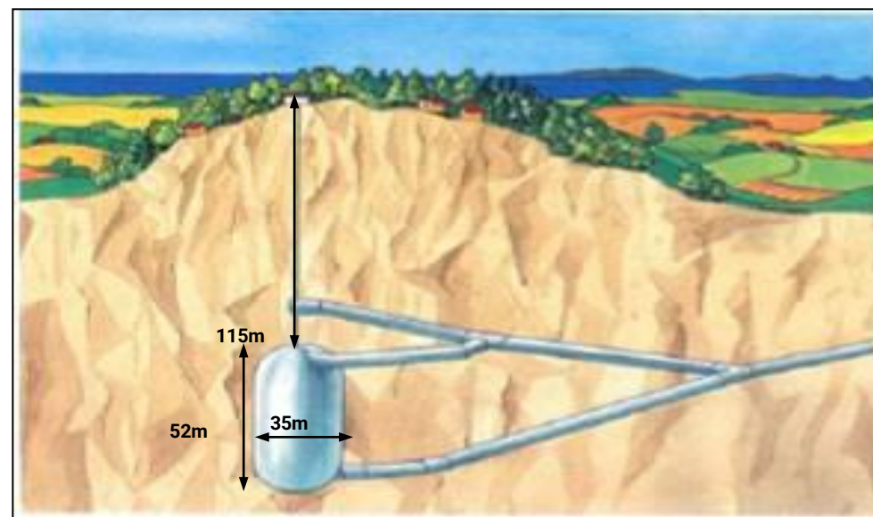
Cavités minées revêtues (Storengy)
