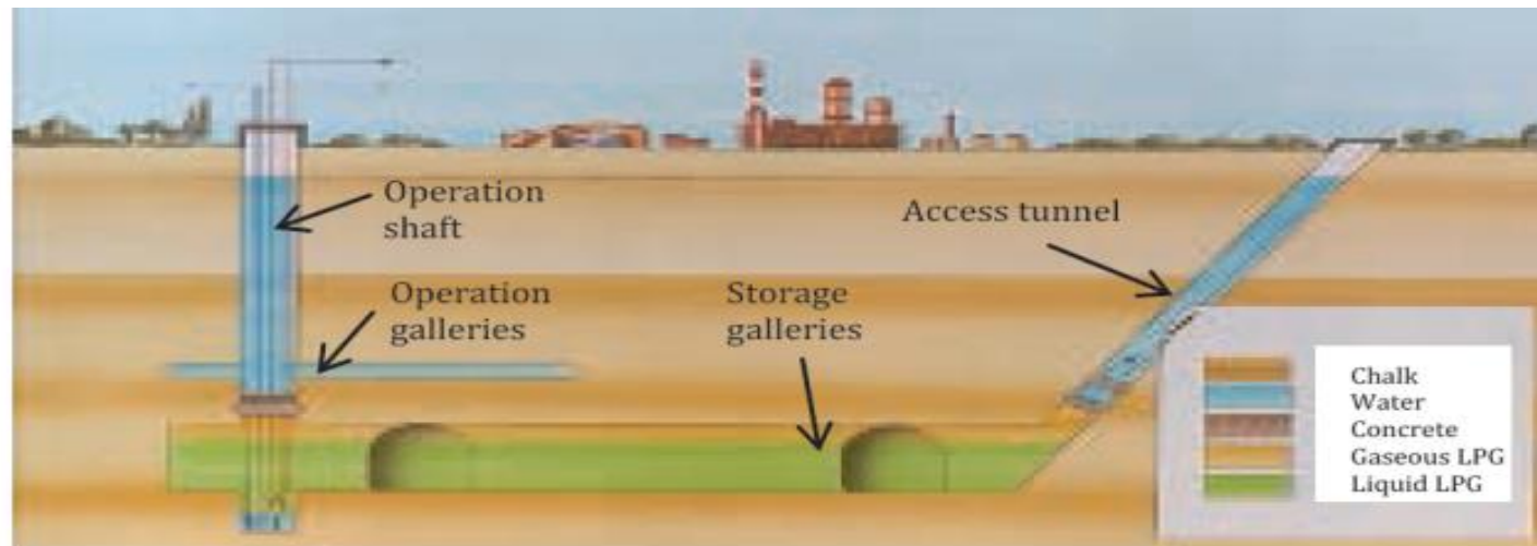
Cavités minées sous barrière hydraulique (Geostock)
