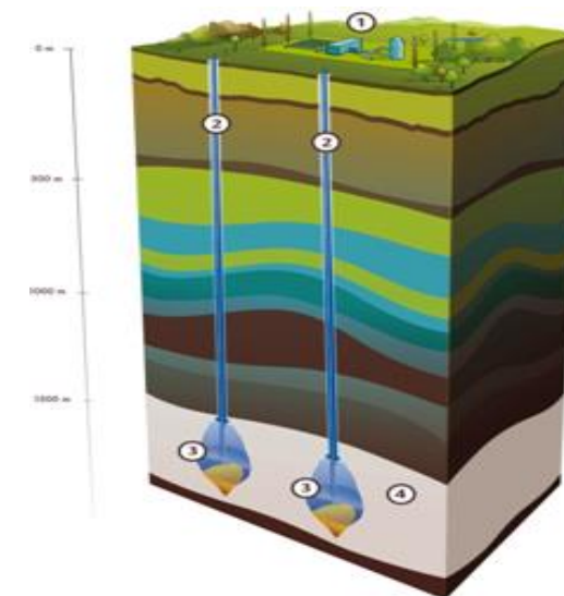
Stockage en cavités salines
