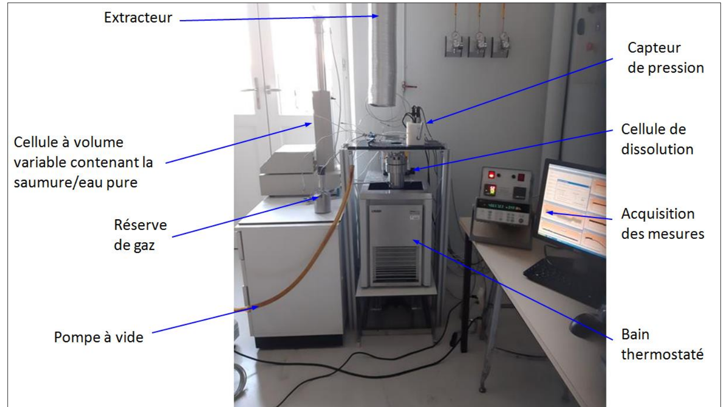
Cinétique de la dissolution
