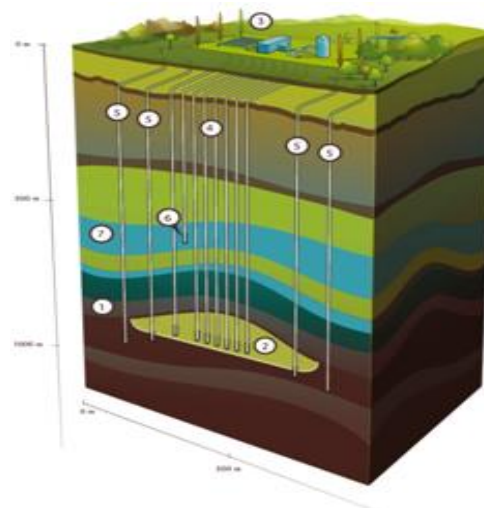
Stockage en nappe aquifère
