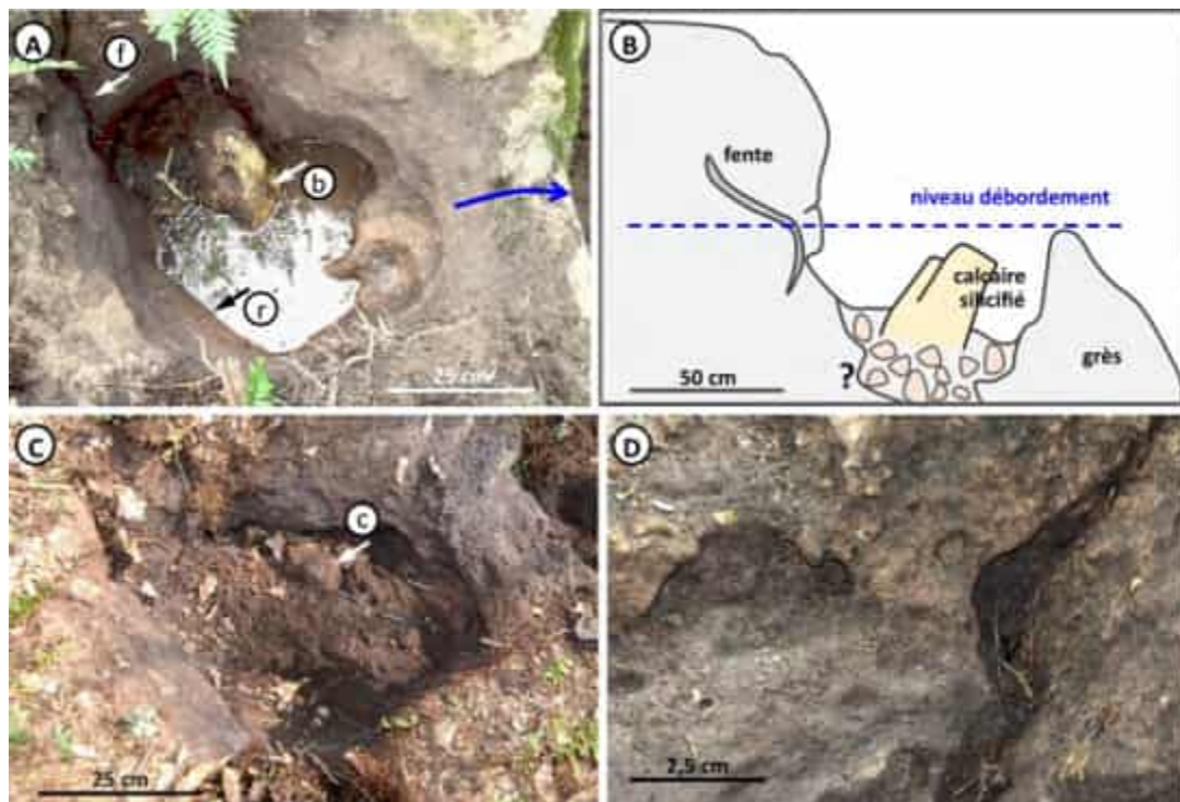
Figure 11 – Le Paradis LPS01 de Courdimanche-sur-Essonne (Essonne). Morphologie du puits. (A) Puits mis à nu par déracinement du châtaignier ; noter le niveau de l'eau de pluie et les morphologies multilobées des parois, la flèche bleue indique le niveau de débordement du puits, (b) un gros caillou figé dans le remplissage, (f) une fente oblique qui s'ouvre dans le puits et (r) paroi rectiligne. (B) Coupe. (C) Puits après remise en place de la terre meuble et cailloux dégagés des racines du châtaignier. (D) fente et paroi dans le haut du puits ; noter le remplissage compact de la fente par des racines ainsi que les alvéoles d'altération à la surface de la paroi.
