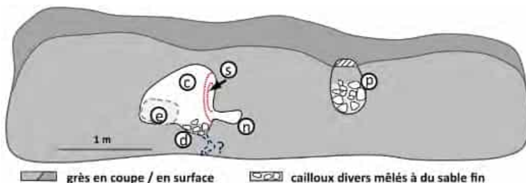
Figure 4 – Le Paradis LPS01 de Courdimanche-sur-Essonne (Essonne). Coupe schématique du bloc avec position des principaux éléments morphologiques. (p) « puits » ; (c) cavité ; (e) entrée ; (s) structure annulaire ; (n) niche ; (d) dépression dans le sol.
