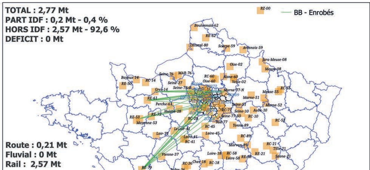
Figure 10 : Carte des flux de granulats pour le BB dans la situation initiale.
