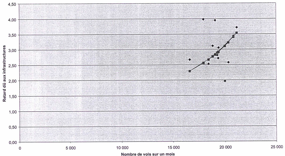
Comparaison modélisation / réalité pour l'aéroport de Roissy en 2002
