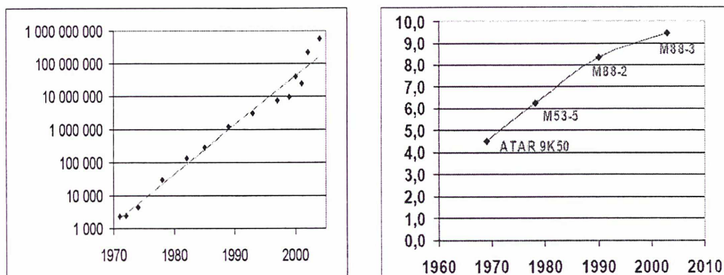
Évolution du rapport poussée sur poids pour un moteur Snecma
