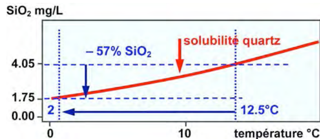
Figure 6 - La solubilité du quartz baisse de plus de la moitié quand la température baisse de 12,5 et 0°C (document Médard Thiry).
