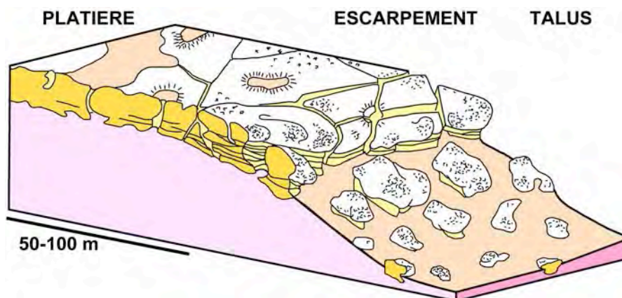
Figure 12 - Schéma de démantèlement des platiers de grès (document Médard Thiry).
