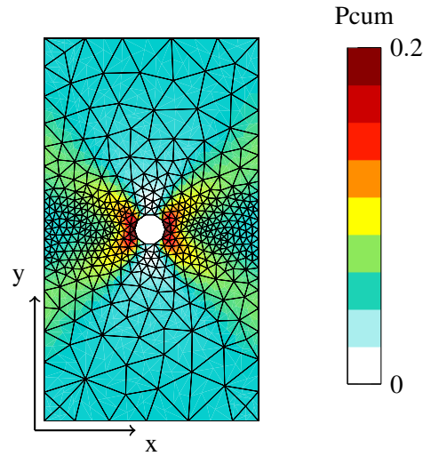
FIGURE 3 – Champ de plasticité cumulée. On note les valeurs non nulles près des bords.
