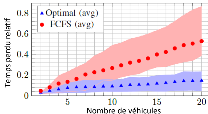
Figure 7 : Gain de temps rendu possible par un ordonnancement optimal des véhicules à une. Lecture : un temps perdu relatif de 1 indique que les véhicules mettent en moyenne deux fois plus de temps à traverser l'intersection qu'il ne leur en faudrait si l'intersection était vide.
