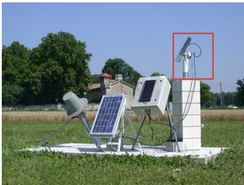
Figure 9 : Station de mesure AERONET, à droite (dans le rectangle rouge), le bras robotisé de mesure et ses équipements pour son apport en énergie et la transmission des données par satellites lorsque cela est possible. (Source : http://aeronet.gsfc.nasa.gov )
