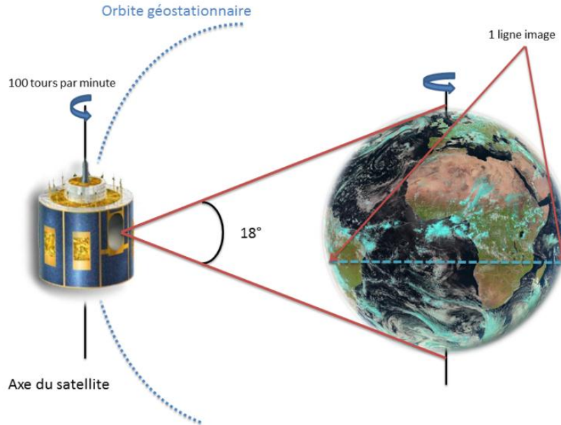
Figure 16 : principe de la mesure de MFG et MSG
