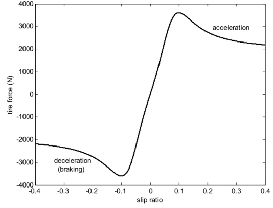
FIGURE 4 – Force longitudinale en fonction du taux de glissement longitudinal
