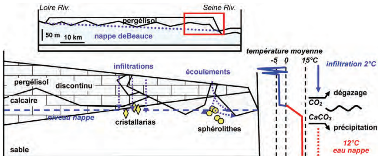
Fig. 32 : Schéma conceptuel de la précipitation des calcites sableuses pendant les périodes froides du Quaternaire. C'est le réchauffement des eaux d'infiltration dans le sous-sol qui induit la précipitation des calcites sableuses dans les aquifères sableux.
