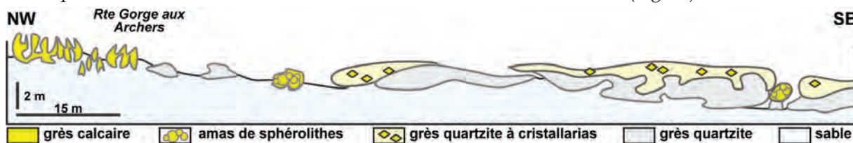
Fig. 12 : Schéma de la disposition des différents faciès de grès calcaire et cristallarias de calcite en bordure de la platière des « Béorlots ».
