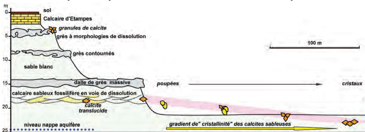
Fig. 14 : Schéma du gisement de calcites sableuses de la carrière des « Gondonnères ». Les sables sont blancs sur toute la hauteur de l'exploitation, des sables jaunâtres apparaissaient par endroits au plancher de la carrière. Une grande variété de calcite sableuse se disposait selon un niveau faiblement incliné qui se raccordait à un niveau coquillé altéré.
