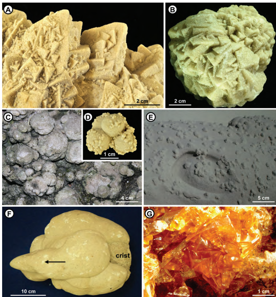
Fig. 2 : Calcites sableuses: (A) grands rhomboédres en gerbes (axes rayonnants) auxquels se superposent de petites pointes de rhomboèdre (Puisselet, 77), échant. 8609 ; (B) cristallaria à rhomboédres enchevêtrés (La Garenne, Darvault, 77), échant. 8931 ; (C) sphérolithes coalescents (Roche à Boule, Montigny/Loing, 77) ; (D) sphérolithes avec petits sphérolithes secondaires (carrière Bonnevault, Larchant, 77) ; (E) grès «clouté» de petits granules de calcite (carrière des Gondonnères, Larchant, 77), idem échant. 8943 ; (F) poupée calcaire englobant une cristallaria à pointes de rhomboèdre (crist) ; la disposition des concrétions successives et leur allongement donne le sens de l'écoulement de l'eau (flèche) qui a précipité la calcite, (carrière des Gondonnères, Larchant, 77) ; (G) cristaux de calcite limpide (carrière des Gondonnères, Larchant, 77), échant. 8787. Les numéros sont ceux des échantillons qui ont été datés (Tab. I). Clichés : M. THIRY, sauf (B) Ph. LE CAER (Mines-ParisTech) et (G) M. BERGER (Mines-ParisTech).
