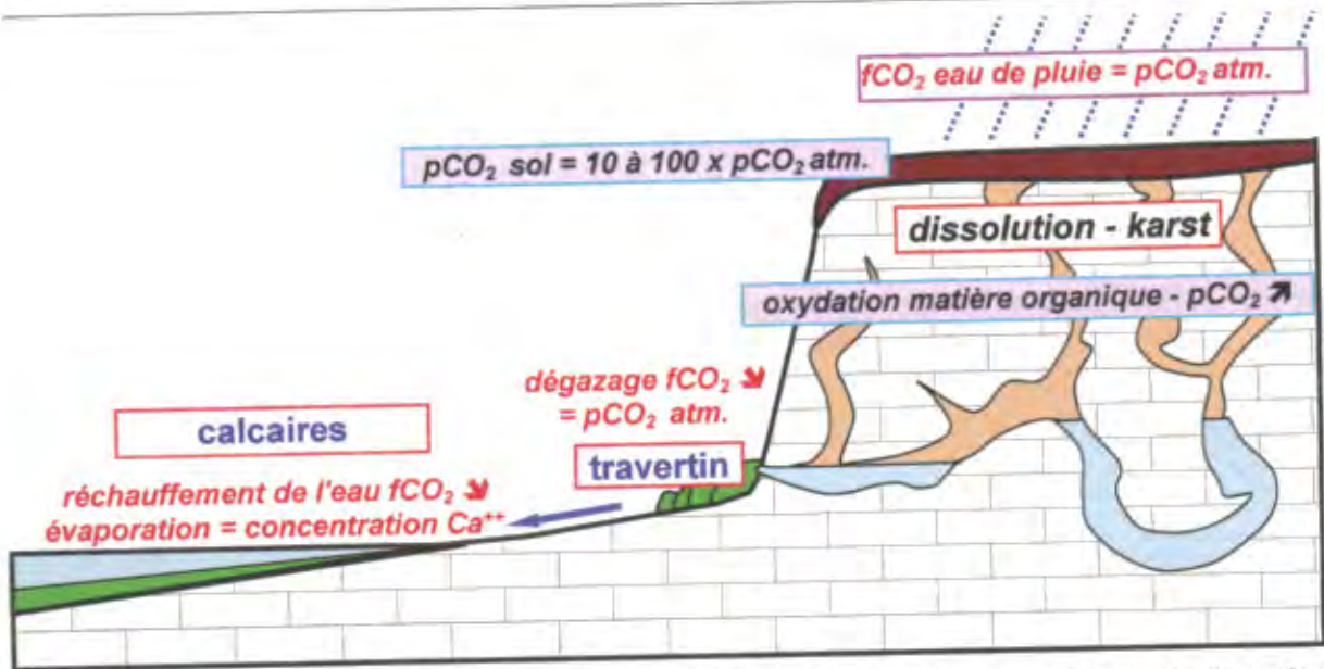
Fig. 4 : Schéma du « cycle » du \text{CO}_2 dans les eaux superficielles et de sub-surface et son effet sur les formations calcaires.
