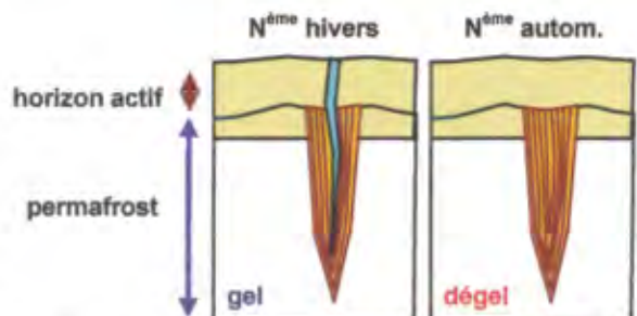
Fig. 16 : Schéma de formation des coins de glace dans les pergélisols.
