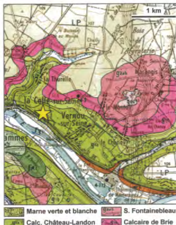
Fig. 8 : Situation du gisement de La Celle-sur-Seine dans son contexte géologique (extrait carte géologique 1/50 000 e - Fontainebleau).
