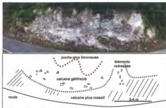
Fig. 14 : Affleurement et schéma interprétatif de l'affleurement cryoturbé visible dans le virage de la côte du Panorama à Champagne-sur-Seine. Les calcaires sont gélfraités et un début d'organisation d'une poche cryoturbée se distingue. Cliché : M. THIRY.
