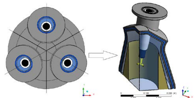
Figure 1 : Vue du dessus et vue 3D du tiers de la torche modélisé
