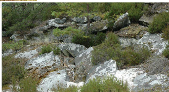
Fig. 12 : Dalle de grès effondrée et fracturée par affouillement éolien en bordure d'une alvéole de déflation bien délimitée. Route Descamps (parcelle 628). Cliché : M. THIRY.
