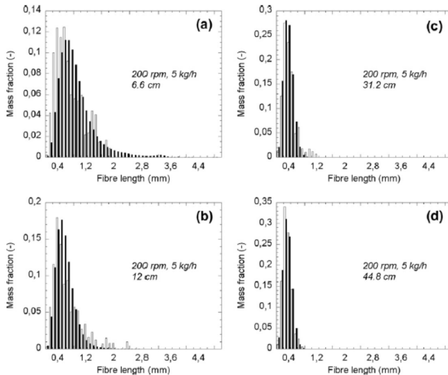
Figure 5. Distribution des longueurs de fibres à différentes positions le long des vis pour une condition d'extrusion fixée. Comparaison entre le modèle (blanc) et l'expérience (noir)
