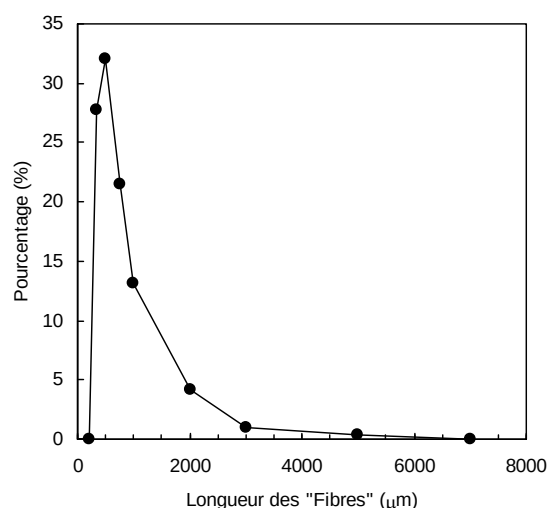
Figure 5. Distribution des longueurs des "Fibres" en sortie de filière (1 kg/h, 200 tr/min, introduction après fusion).
