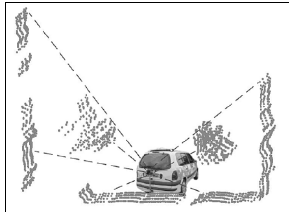
Figure 2 Fonctionnement du scanner laser par profil
