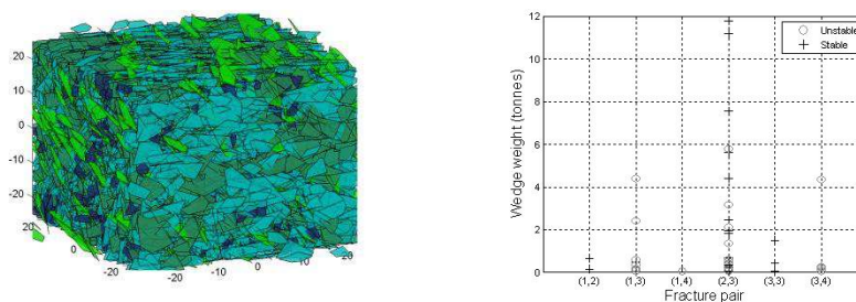
Figure 1. Utilisation d'un DFN pour établir les instabilités structurales potentielles le long d'un talus rocheux, [GRE 08].
