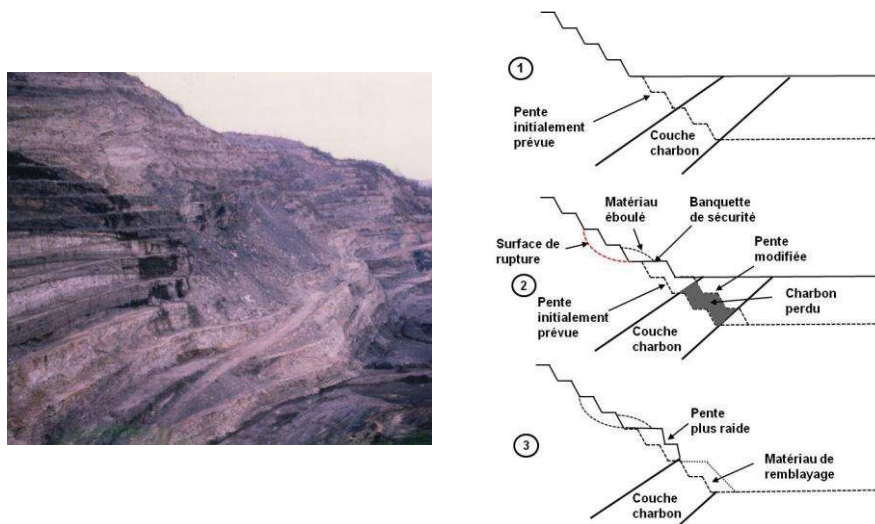
Figure 4 : Flanc ouest de la mine de charbon de Decazeville: vue générale et instabilité de pente (gauche) et gestion des travaux d'excavation (droite) [COJ 01]
