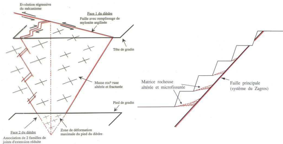
Figure 7. Mécanismes de glissement plan ou en dièdre cinématiquement possible seulement si le massif rocheux fortement altéré et fissuré peut se déformer ou se rompre.
