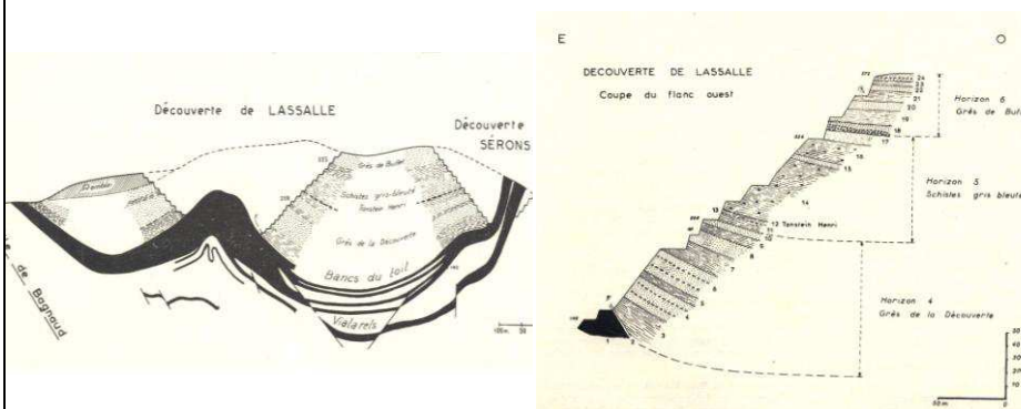
Figure 3 : Coupe NE-SW de la découverte de Lassalle et de Sérons (gauche) et du flanc ouest de la découverte de Lassalle, [VET 68]
