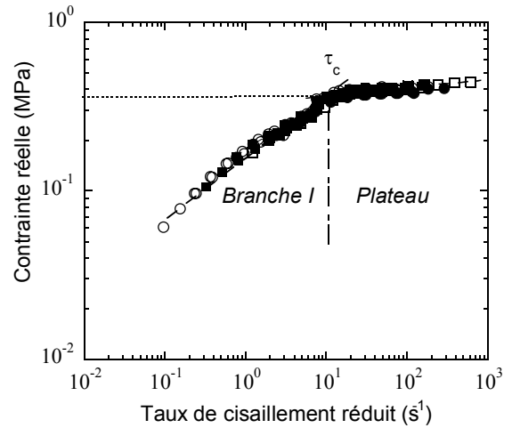
Figure 2. Courbe maîtresse à T_{ref} = 70^\circ\text{C} obtenue par superposition temps-température ( \bullet 40^\circ\text{C} , \square 50^\circ\text{C} , \blacksquare 70^\circ\text{C} , \circ 90^\circ\text{C} )
