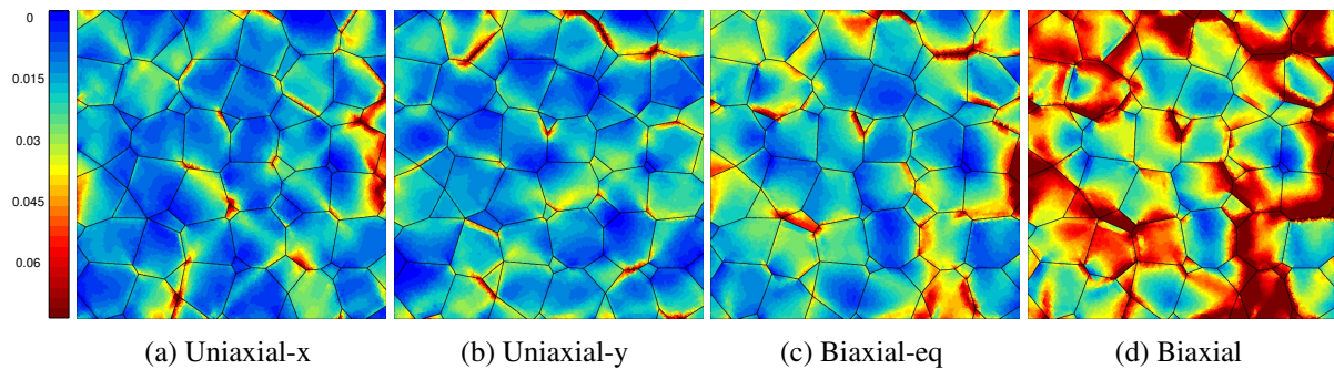
Fig. 3 – Carte de la somme des glissements cumulés \sum \gamma_{cum} en surface libre sous différents chargements.
