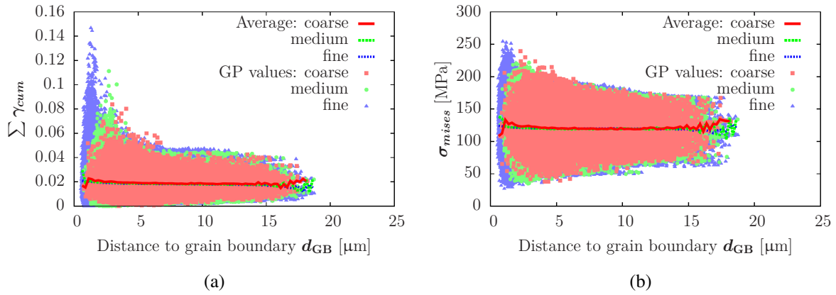
Fig. 2 – Déformation plastique \sum \gamma_{cum} et de contrainte de von Mises \sigma_{mises} en fonction de la distance aux joints de grains pour différents densité de maillage. Sont tracées à la fois les valeurs discrètes aux points de Gauss (points en couleurs claires) et la moyenne par tranche (en courbes foncées).
