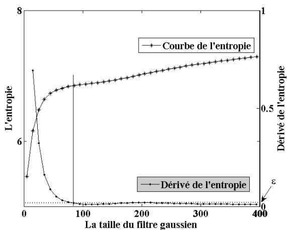
Figure 2 : Courbe d'entropie montrant une diminution de la pente quand la taille du filtre gaussien est supérieure au plus grand objet de l'image
