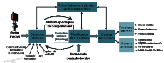
Figure 1 : Schéma fonctionnel
