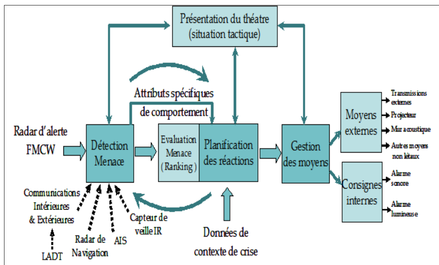
Figure 1. Schéma fonctionnel du système SARGOS
