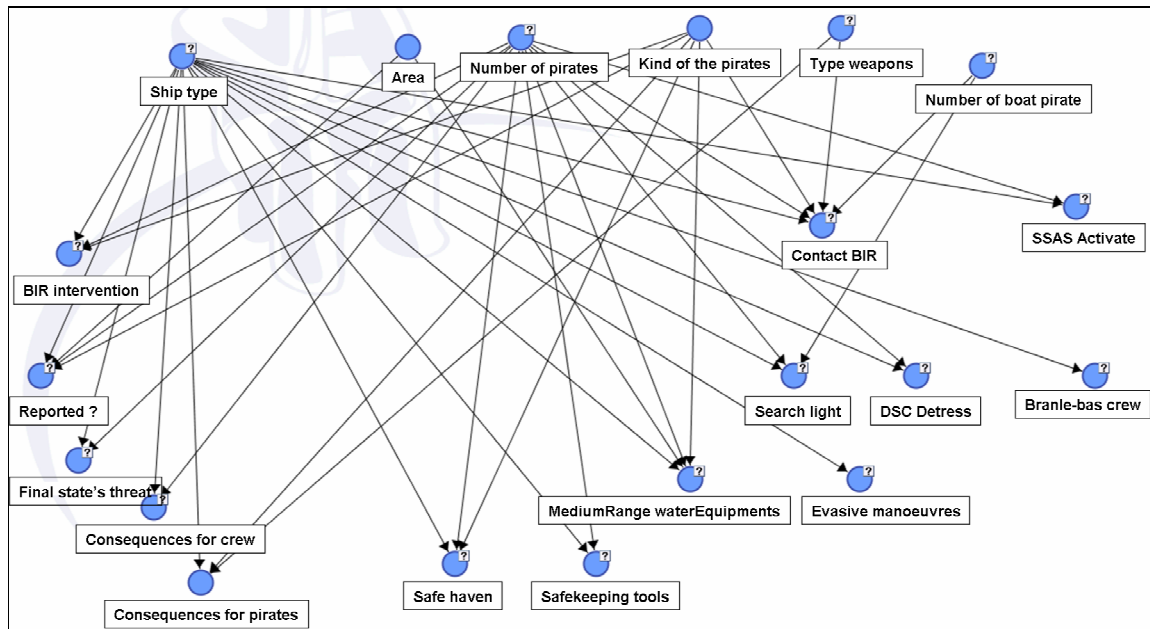
Figure 2. Réseau bayésien basé sur les données OMI
