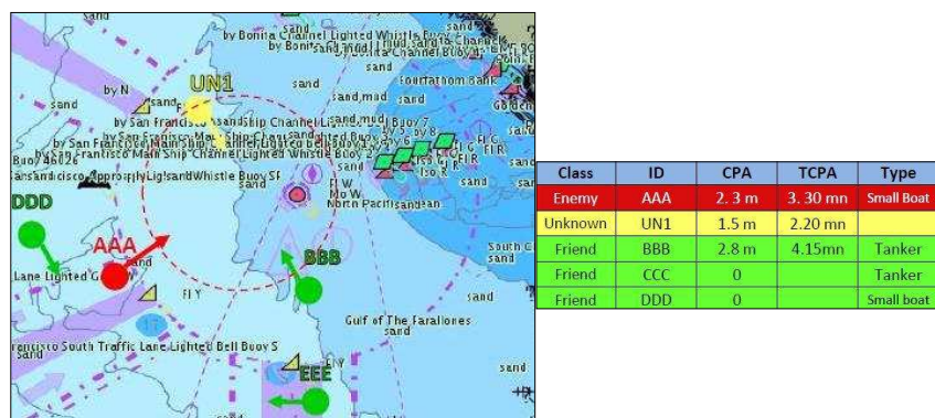
Figure 7. Hiérarchisation des menaces dans l'interface Homme-Machine du système SARGOS
