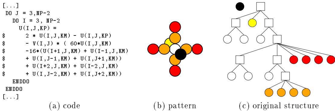
Figure 4: ONDE24 kernel.
