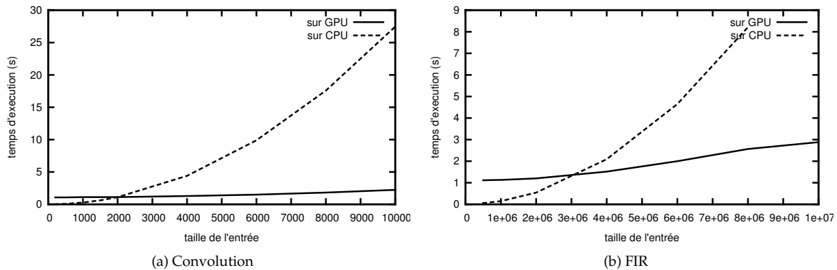
FIGURE 7 – Temps d’exécution sur GPU pour des noyaux de traitements d’images générés par p4a.
