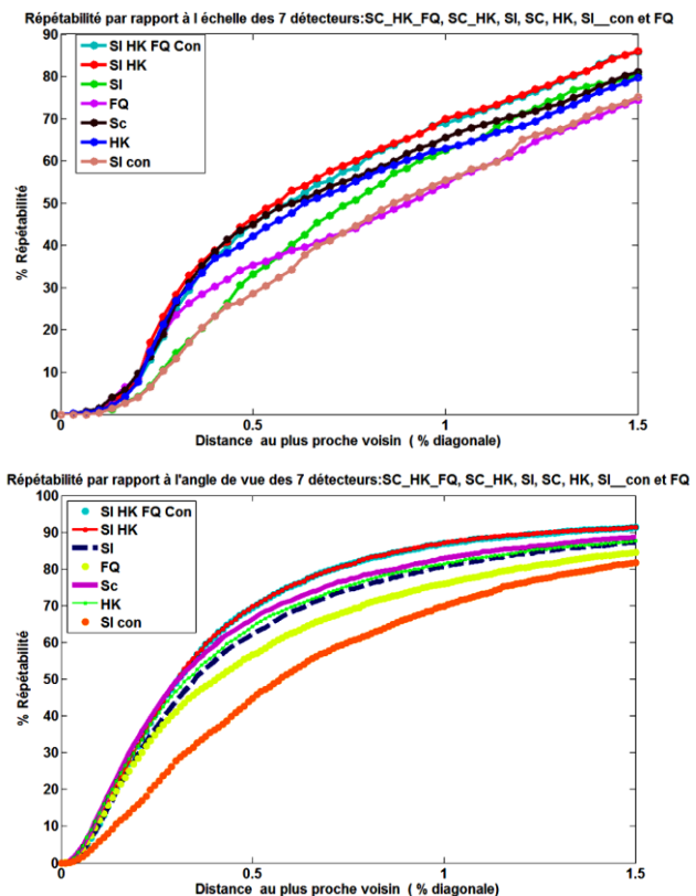
Figure 4. Répétabilité des 7 détecteurs testés pour les objets de la base Minolta en fixant le nombre le keypoint. En haut, à un changement d'échelle pour 2 objets avec 55 vues- en bas, à une variation de l'angle de vue (293 angles de vues) pour 15 objets. Seulement la partie gauche des graphes obtenus est représentée.
