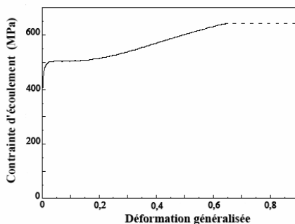
a) Courbe d'érouissage du métal- Stress-strain curve of the metal
