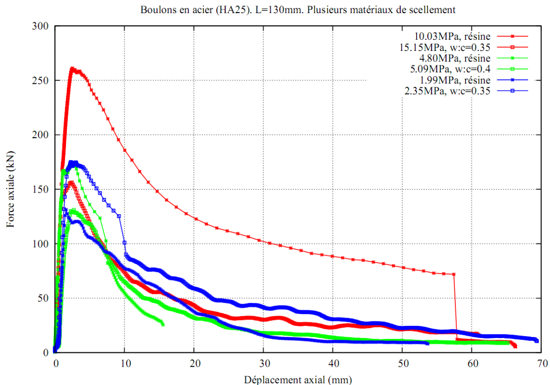
Figure 15 : Essais d'arrachement sur les boulons HA25. L=130\text{mm} . Scellements différents
