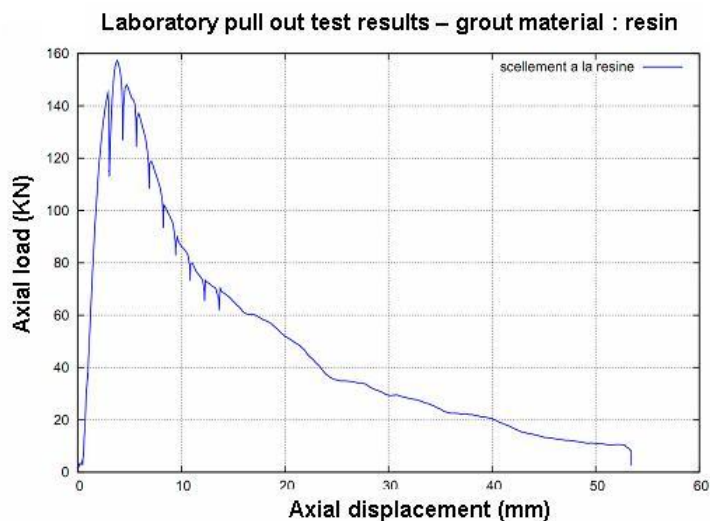
Figure 10 : Résultat de l'essai d'arrachement pour L=150mm, P=5MPa, scellement à la résine
