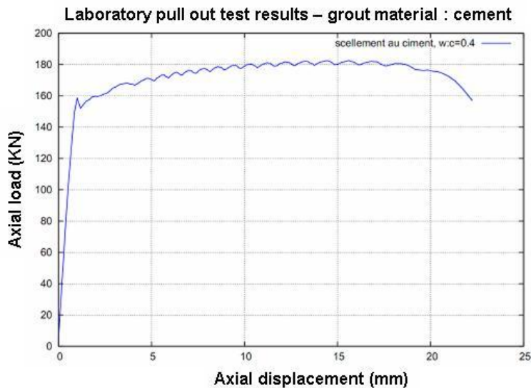
Figure 9 : Résultat de l'essai d'arrachement pour L=300mm, P=15MPa, w:c=0,4
