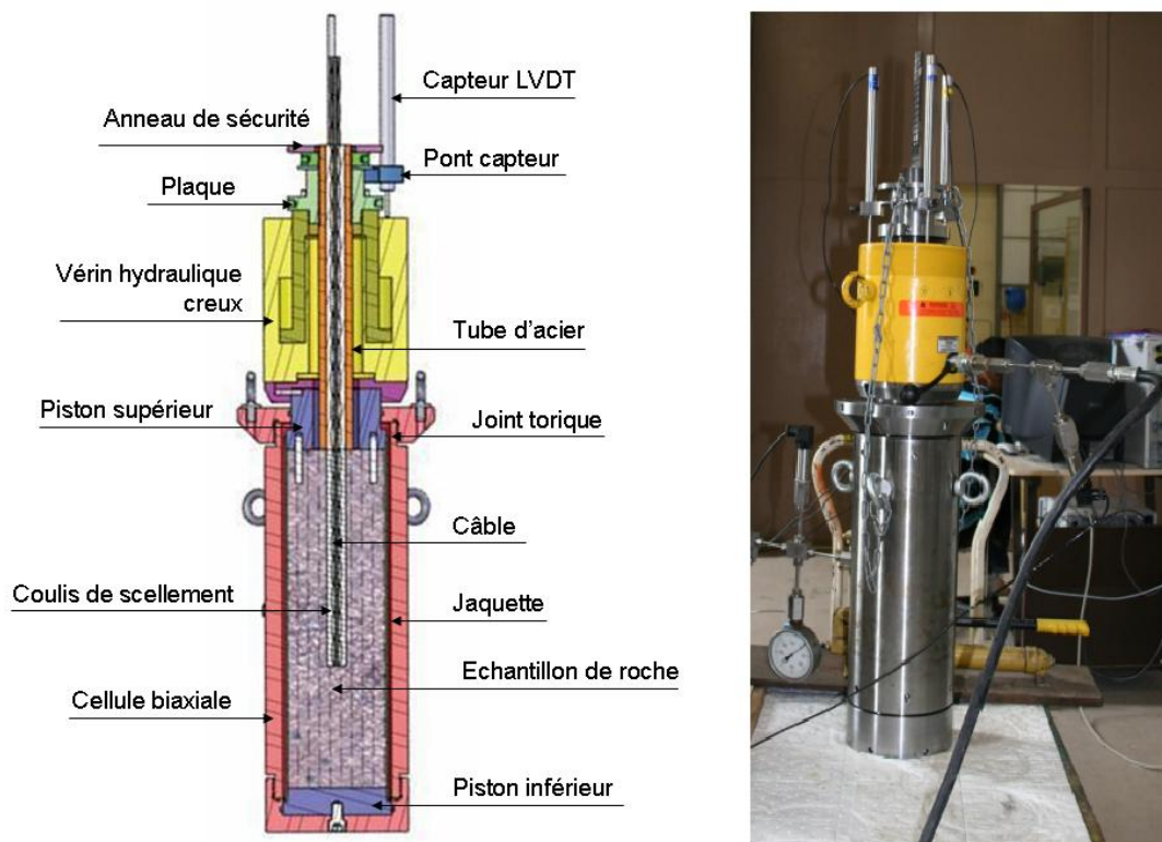
Figure 7: principaux éléments du banc expérimental et vue pendant un essai
