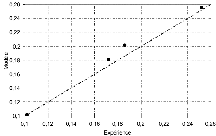
FIG. 5 – Comparaison entre la ténacité modélisée et expérimentale
