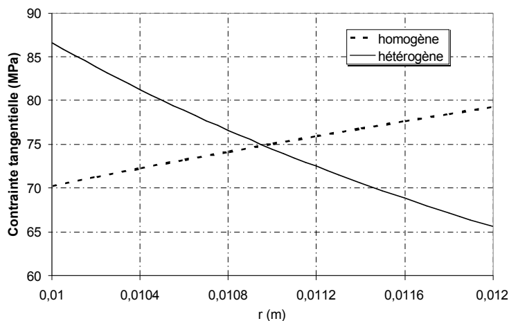
b. Distribution de la contrainte tangentielle
