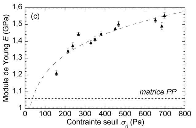
Figure 4 : Rapport d'aires A_r (a) et contrainte seuil \sigma_0 (b) en fonction de l'EMS, module de Young en fonction de la contrainte seuil (niveau d'exfoliation) (c)
