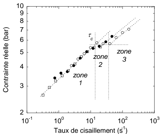
Fig. 6 : Evolution de la contrainte réelle en fonction du taux de cisaillement apparent (SBR chargé, diamètres 2 mm (□), 3 mm (◻) et 4 mm (◻), 70°C)
