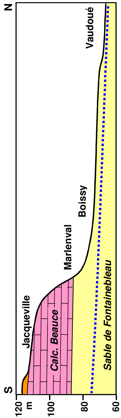
Figure 3 – Coupe géologique le long de la vallée de l'École. La rupture topographique en fond vallée est due à l'escarpement du Calcaire de Beauce. Le saut topographique au sud du Vaudoué n'a apparemment pas de rapport avec un changement lithologique. Il serait dû à un ancien barrage ? La nappe phréatique est à environ 3 à 5 m de profondeur dans la vallée sèche de Marlival – Boissy aux Cailles.
