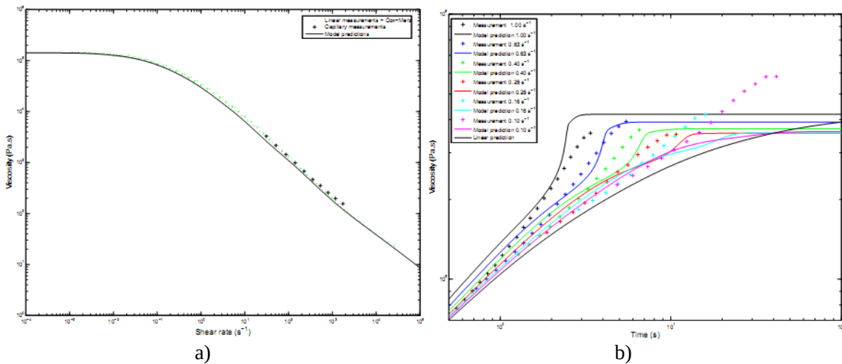
Figure 3 : Confrontation experience/modèle : (a) rhéologie en cisaillement ; (b) rhéologie élongationnelle
