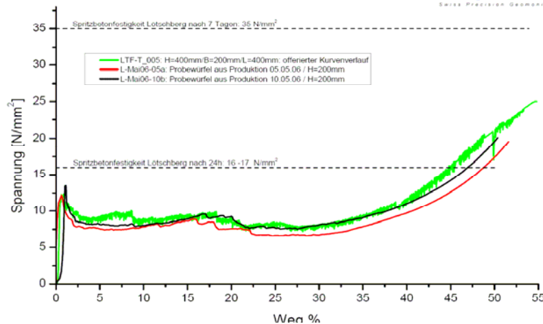
Fig. 22 : Courbe de l'essai en compression simple des blocs compressibles
