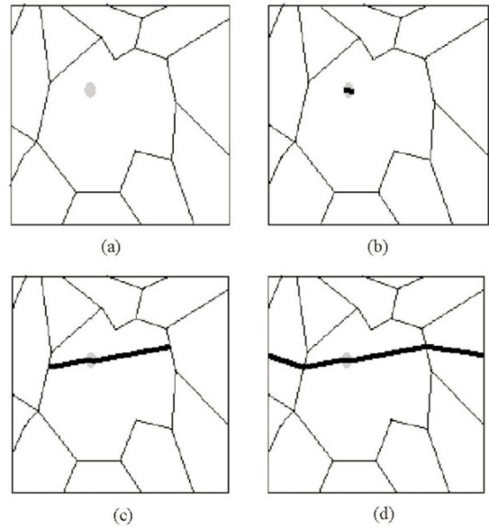
Fig. 4 へき開破壊に及ぼす微視組織学的障壁の効果の模式図：a) 損傷前, b) 粒子における微視き裂生成, c) 粒子/マトリックス界面を横切る微視き裂伝播とパケット境界での停留, d) 最終破壊につながるパケット境界を横切るき裂進展 2)
