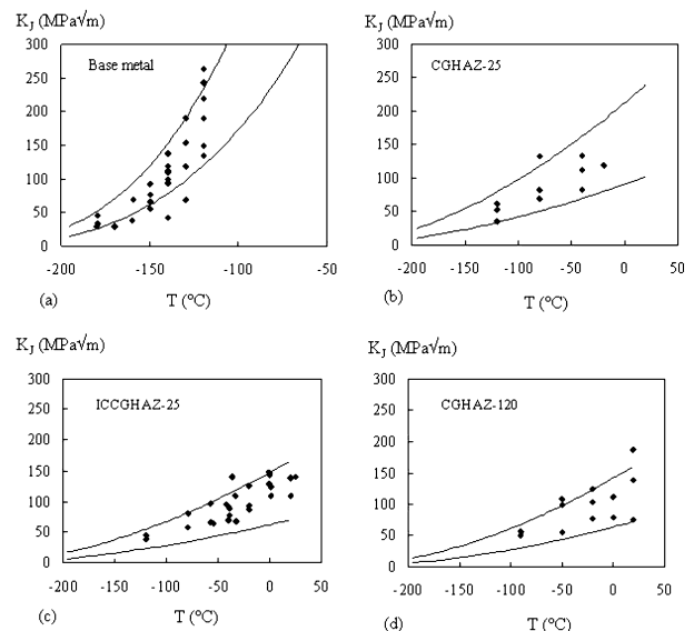
Fig. 9 再現 HAZ における破壊靱性の温度依存性。実験結果（プロット）と累積破壊確率 10% および 90% に対応する Beremin モデルの予測値（2つの曲線）を比較したものである。a) 母材, b) CGHAZ-25s, c) ICCGHAZ-25s, d) CGHAZ-120s, 25s あるいは 120s という数字は、800~500 度の冷却時間 (秒) を示している 4, 9 。
