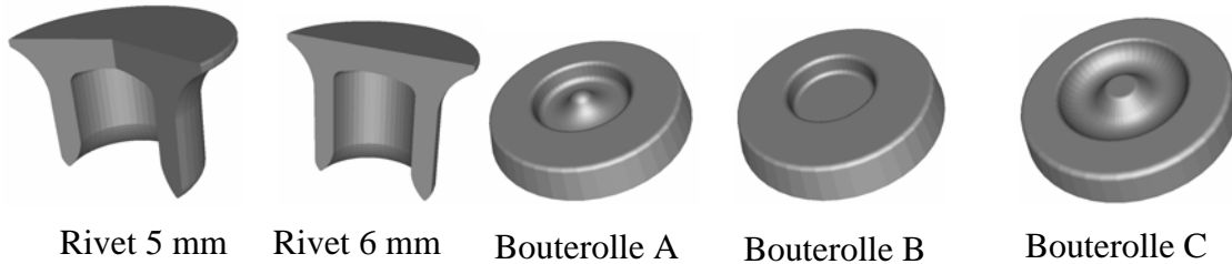
Figure 2 - Géométrie des rivets et bouterolles
