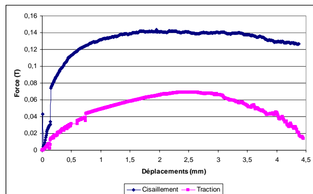
Figure 9 – Courbes Efforts-Déplacements pour l'essai de cisaillement et de traction
