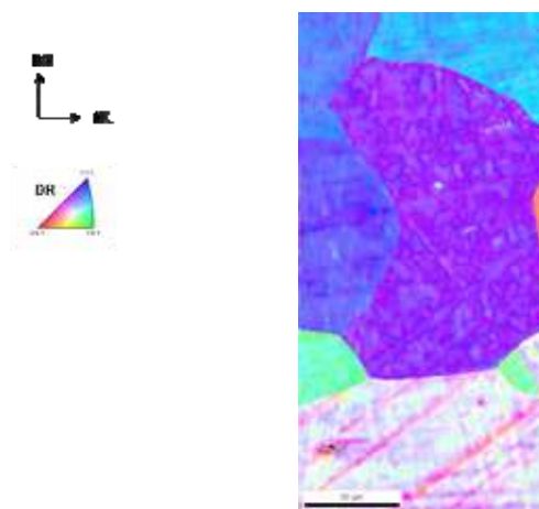
Figure 14. Microstructure après recuit sur la zone fluotournée
