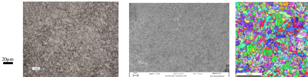
Figure 2 : microscopie optique (à gauche), image MEB (au centre), cliché EBSD (à droite) du métal de base. L'échelle est elle vraiment la même pour ces trois figures ?
