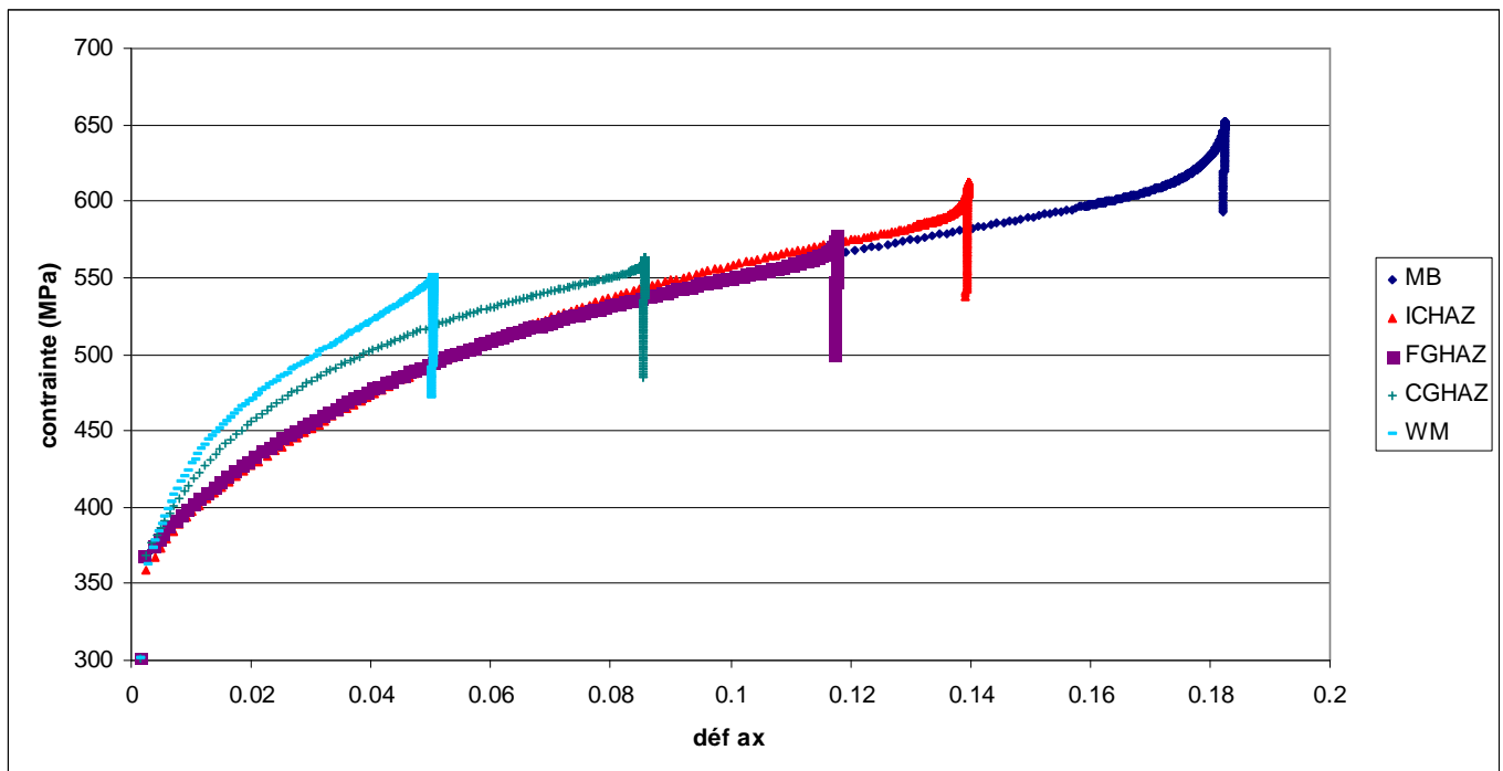
Figure 12 : courbes de traction des différentes zones du joint soudé après calcul éléments finis
