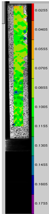
Figure 17 : champ de déformation axiale dans une éprouvette de métal de base avant striction, pour une déformation nominale de 13.5%
