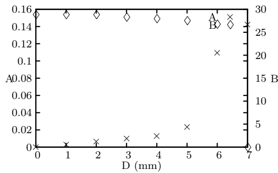
FIG. 4 – Détection des ruptures de fibres dans le composite carbone/époxy. Epreuve de 3 mm d'épaisseur. Corrélation entre la perte de pente (B) de la courbe de flexion en fonction de la flèche de flexion maximale atteinte ( D , unité : mm) et l'amplitude de \frac{\Gamma-\Gamma_R}{\Gamma_R} (A) en fonction de la flèche de flexion maximale atteinte mesurée aux retours à un déplacement nul. Mesures à la fréquence de résonance 570 MHz.
