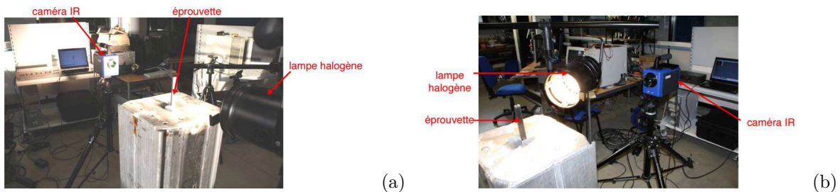
FIG. 10 – Dispositif expérimental de thermographie infrarouge. (a) Cas de la transmission. (b) Cas de la réflexion.
