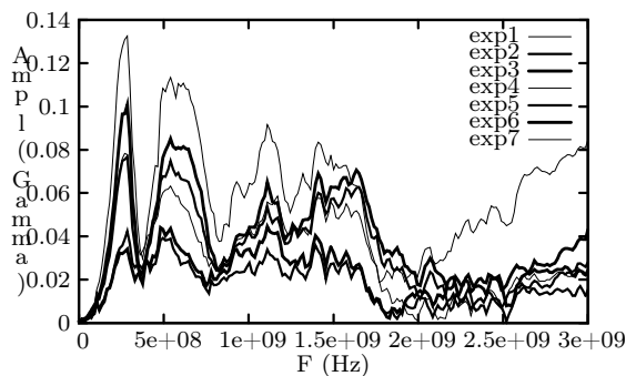
FIG. 6 – Détection des ruptures de fibres dans le composite carbone/époxy. Epreuve de 8 mm d'épaisseur. Amplitude de \frac{\Gamma-\Gamma_R}{\Gamma_R} (sans unité) en fonction de la fréquence ( F , unité : Hz) aux retours à un déplacement nul. (exp i : mesure après un déplacement maximum atteint de i/2 mm).
