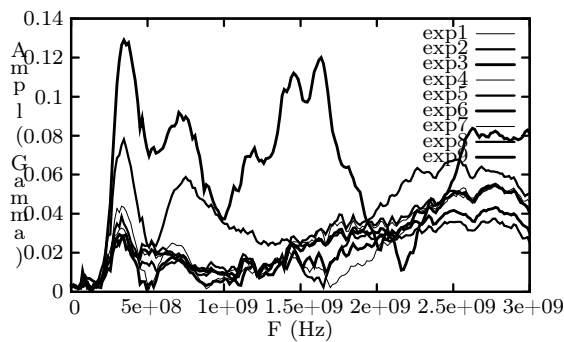
FIG. 5 – Détection des ruptures de fibres dans le composite carbone/époxy. Epreuve de 6 mm d'épaisseur. Amplitude de \frac{\Gamma-\Gamma_R}{\Gamma_R} (sans unité) en fonction de la fréquence ( F , unité : Hz) aux retours à un déplacement nul. (exp i : mesure après un déplacement maximum atteint de i/2 mm).
