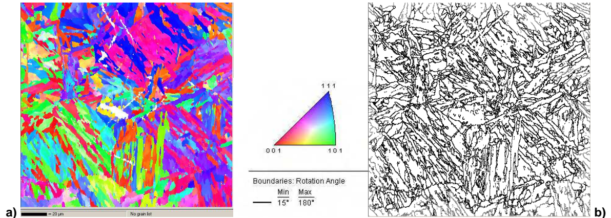
Figure 9: Cartographie d'orientations EBSD a) et cartographie des joints (désorientation >5°) b) de la zone intercritrique.
