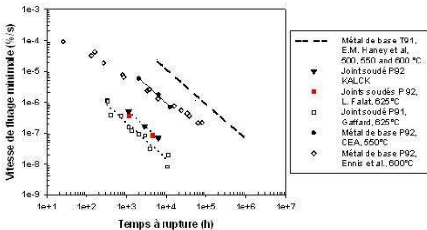
Figure 13 : Courbes de Monkman-Grant du métal de base et de joints soudés Grade 91 et Grade 92 [2, 4, 13, 14].
