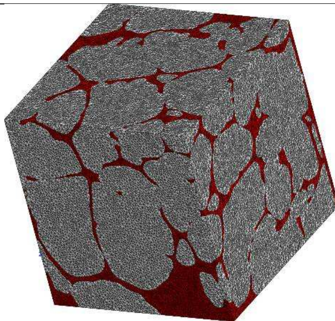
Fig. 6 Exemple du maillage (Volume blanc : zircon ; volume rouge : verre)
