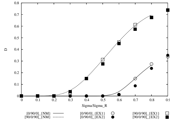
FIG. 2 – Densité de fissuration intralaminaire (sur la totalité du volume de l'éprouvette) détectée par émission acoustique dans la zone d'écoute ( D , nb/mm^3 ) en fonction de la contrainte normée longitudinale appliquée et identification. Les symboles indiquent les points expérimentaux, les lignes continues ou discontinues indiquent l'identification réalisée pour le modèle de fissuration.
