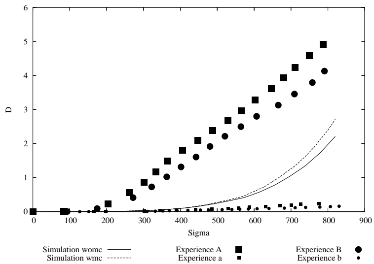
FIG. 6 – Densité de ruptures de fibre (sur la totalité du volume de l'éprouvette) ( D , nb/mm^3 , Expérience A/B : évènements détectés dans la zone d'écoute, Expérience a/b : évènements détectés dans la zone d'écoute et localisés, wmc : simulation avec prise en compte de la fissuration intralaminare, wmc : simulation sans prise en compte de la fissuration intralaminare) en fonction de la contrainte longitudinale appliquée ( \Sigma , MPa ) avec prise en compte ou non du phénomène de fissuration intralaminare. Comparaison entre la simulation et la détection par émission acoustique. (a) (0^\circ_2, 90^\circ_4, 0^\circ_2) (b) (90^\circ_2, 0^\circ_4, 90^\circ_2)
